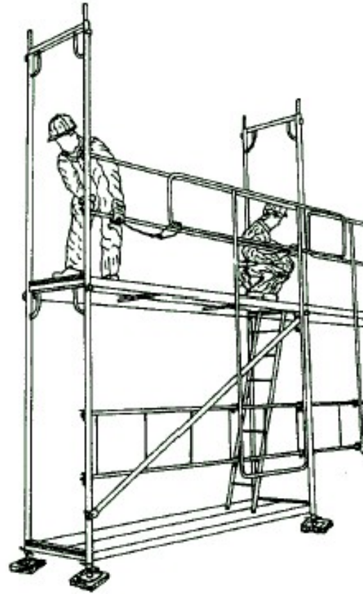
Figura 19. Montaje del resto del andamio
