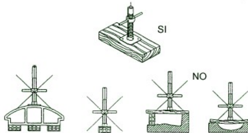
Figura 23. Apoyo correcto e incorrecto de los andamios
