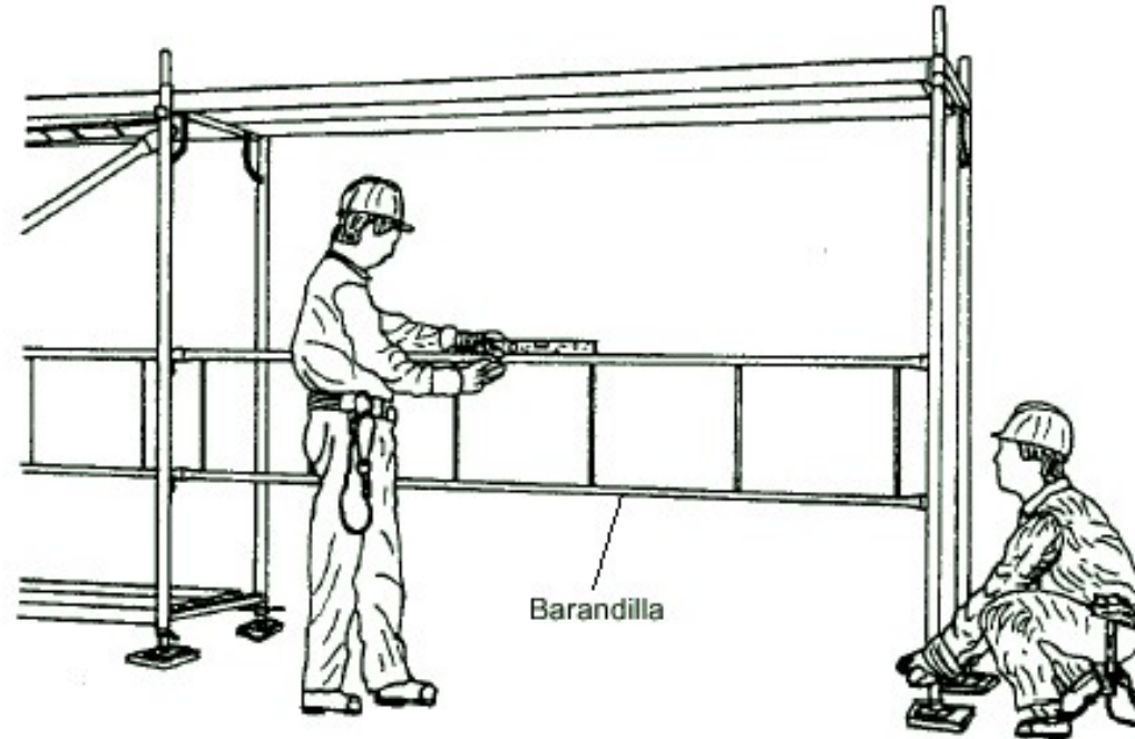
Figura 17. Nivelación horizontal de las barandillas
