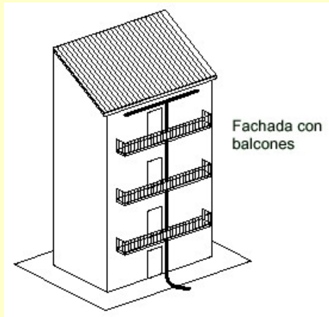
Fig. 25. Distintos casos de instalación de cables de vida en diferentes tipos de edificios
