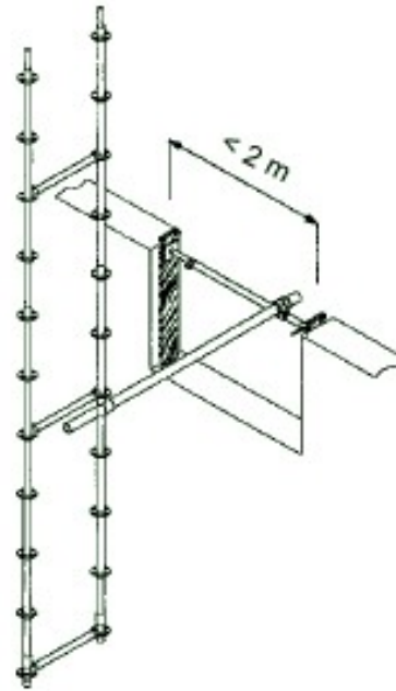
Amarre de ventana Amarre a barra en marco de ventana
