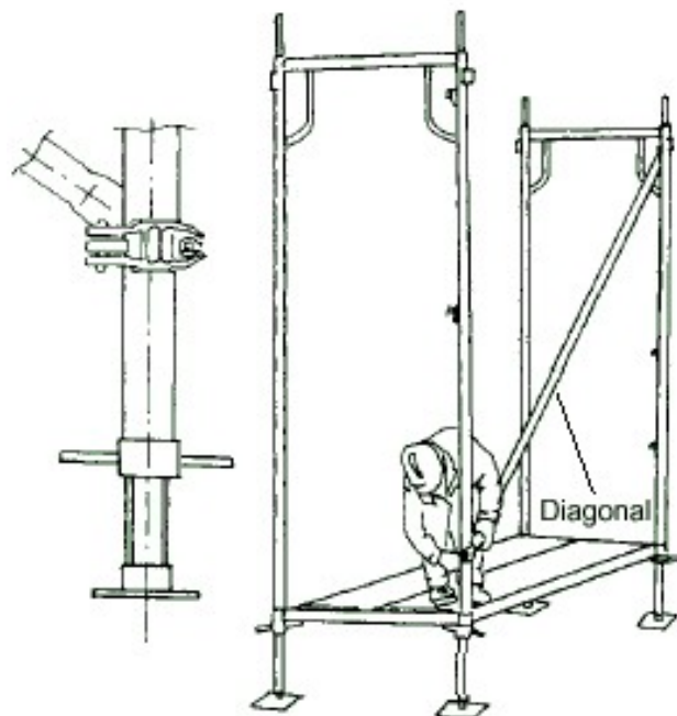
Figura 10. Colocación de los arriostros horizontales diagonales
