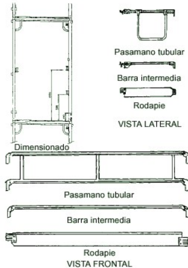
Figura 3. Barandilla de seguridad. Dimensionado
