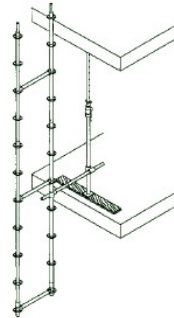
Amarre con puntal metálico
