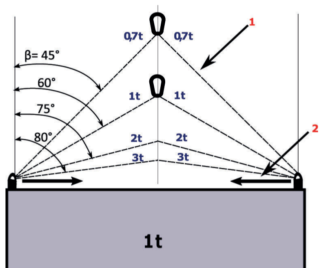
Figura 12. Carga "abrazada" con eslingas cortas, formando un ángulo excesivo con respecto a la vertical. Las eslingas se pueden deslizar por debajo de la carga.
