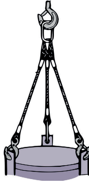
Figura 8. Los puntos de enganche al equipo de elevación y de prensión de la carga aseguran un reparto equilibrado de la carga.
