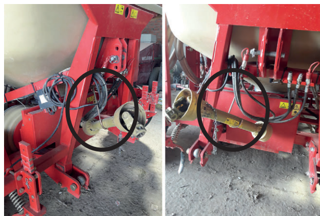
Figura 3. Ejemplo de sistema de sujeción para evitar daños en elementos de transmisión de energía.
