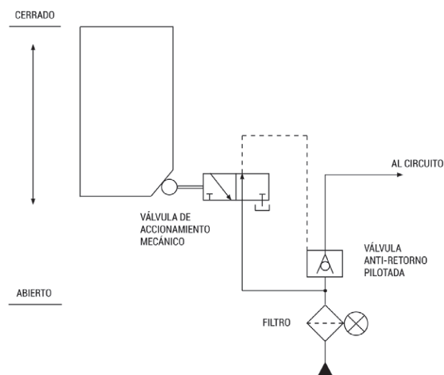
Figura 8. Ejemplo de maniobra de categoría 1 para el enclavamiento entre un resguardo móvil y un accionador hidráulico (maniobra parcial).
