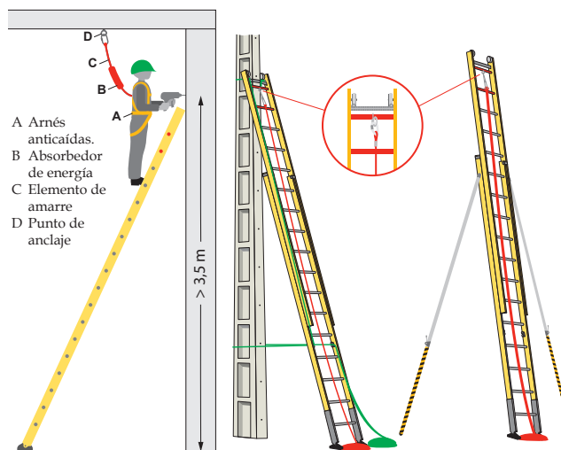
Figura 30. a) utilización de un sistema anticaídas en una escalera de mano. b) escalera con punto de anclaje.
