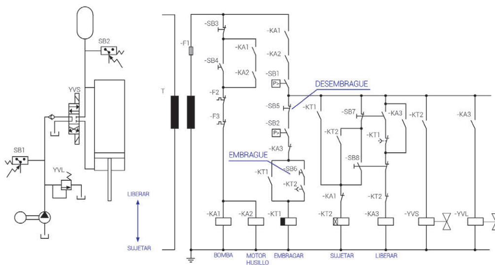
Figura 2. Ejemplo de circuito hidráulico para evitar la pérdida de sujeción de una pieza en un torno. 62
