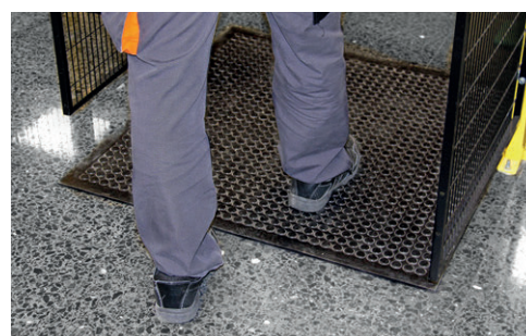
Figura 13. Alfombra sensible. 82
