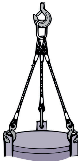
Figura 8. Los puntos de enganche al equipo de elevación y de prensión de la carga aseguran un reparto equilibrado de la carga.
