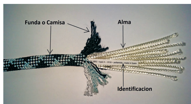
Figura 48. Ejemplo de composición de una cuerda de tipo A.
