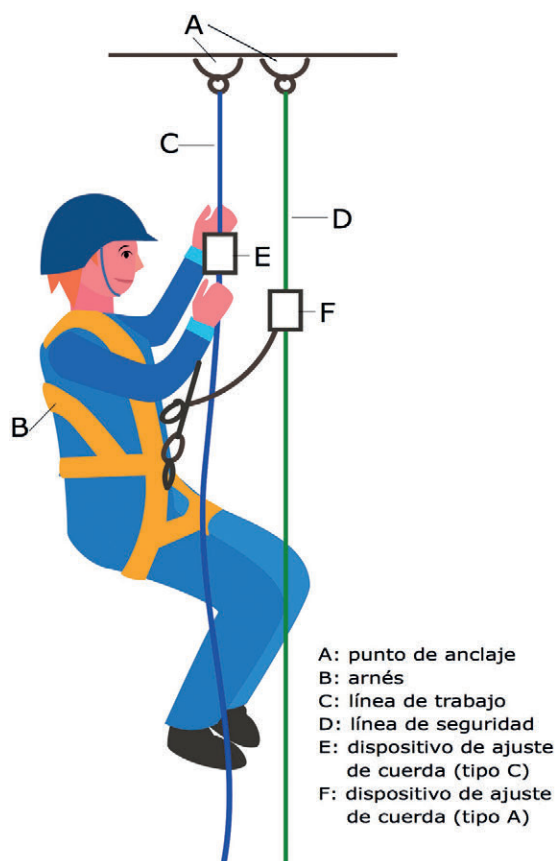
Figura 46. Ejemplo de sistema para el acceso y posicionamiento mediante cuerdas.
