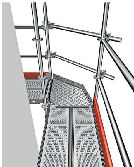
Figura 45. Ejemplo de huecos a cerrar en plataformas.
