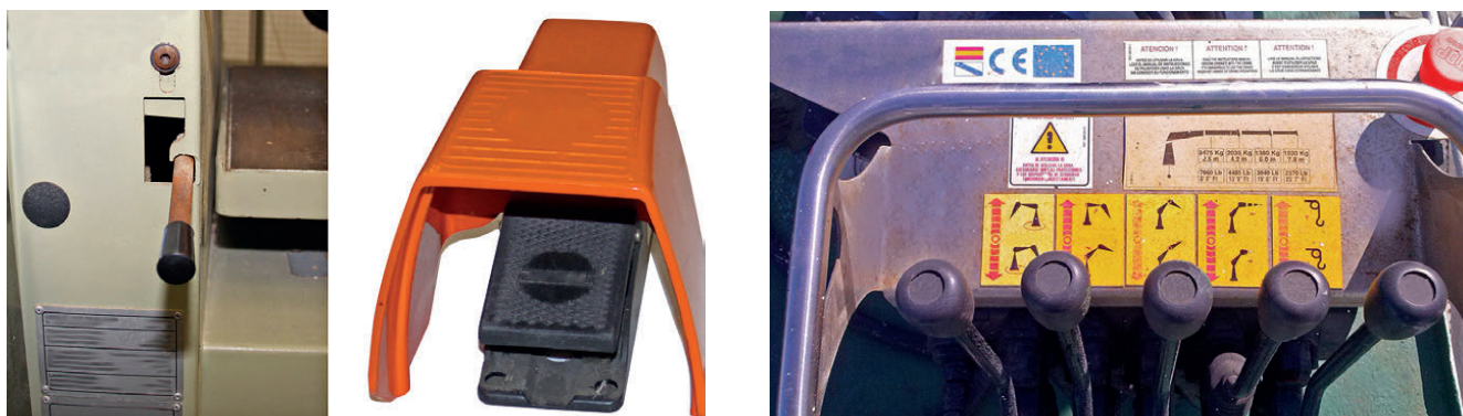
Figura 1. Ejemplos de órganos de accionamiento protegidos contra un accionamiento involuntario.
