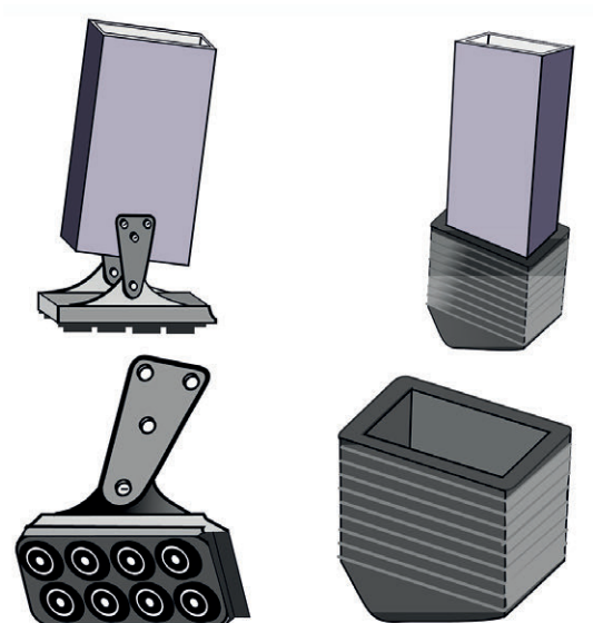
Figura 26. Inmovilización de la parte inferior de una escalera de mano mediante zapatas.
