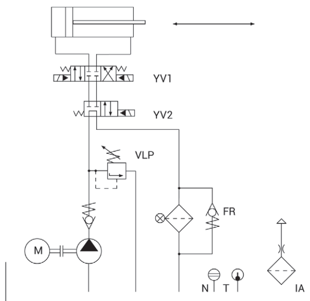
Figura 12. Ejemplo de maniobra de categoría 3 para mando de un cilindro hidráulico (maniobra parcial).
