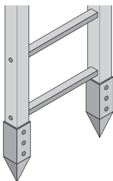
Figura 27. Inmovilización de la parte inferior de una escalera de mano mediante hincas.
