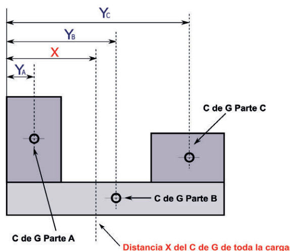
Figura 2. Ejemplo de carga asimétrica.
