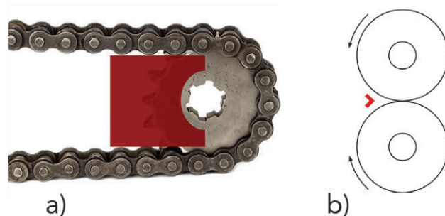
Figuras 1a) y 1b) – Resguardo fijo como protección local. 71
