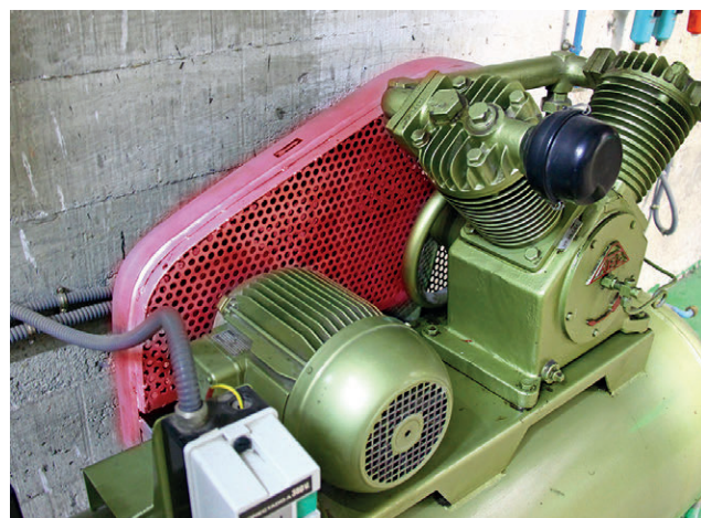
Figura 2. Resguardo fijo envolvente aislando una zona peligrosa. 72
