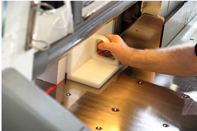
Figura 4: Elemento auxiliar tipo empujador para el talonado/calibrado de la resma
