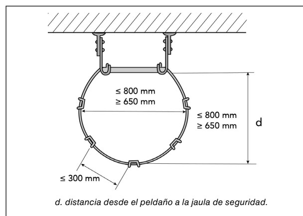
Figura 4. Distancias libres en el interior de una jaula de seguridad
