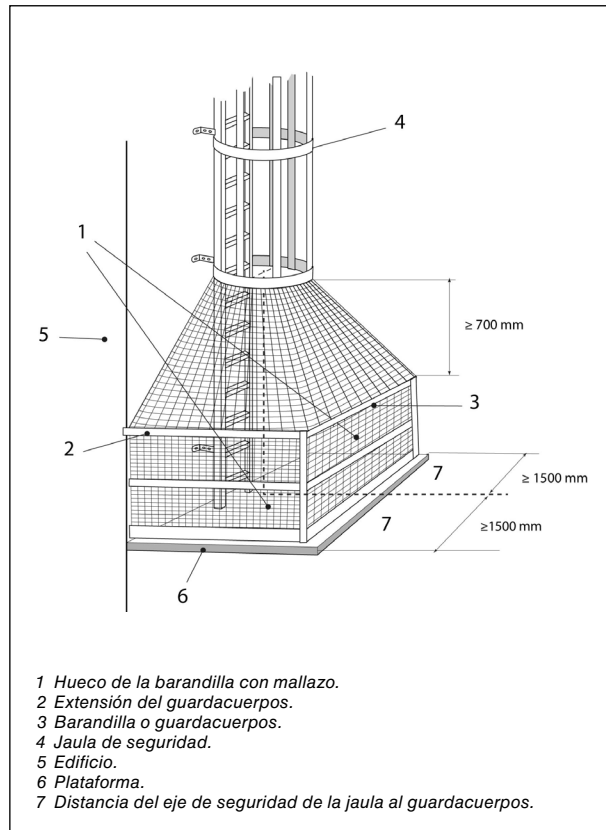
Figura 7. Medidas adicionales al uso de guardacuerpos: estructuras malladas en huecos aéreos y en los huecos del guardacuerpo.
