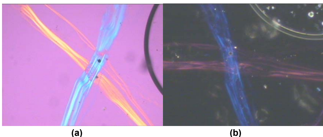
Figura 2. Determinación mediante Microscopía Óptica de (a) carácter cristalino de las fibras seleccionadas mediante polarización y (b) de la variedad de amianto (crisotilo) mediante dispersión.
