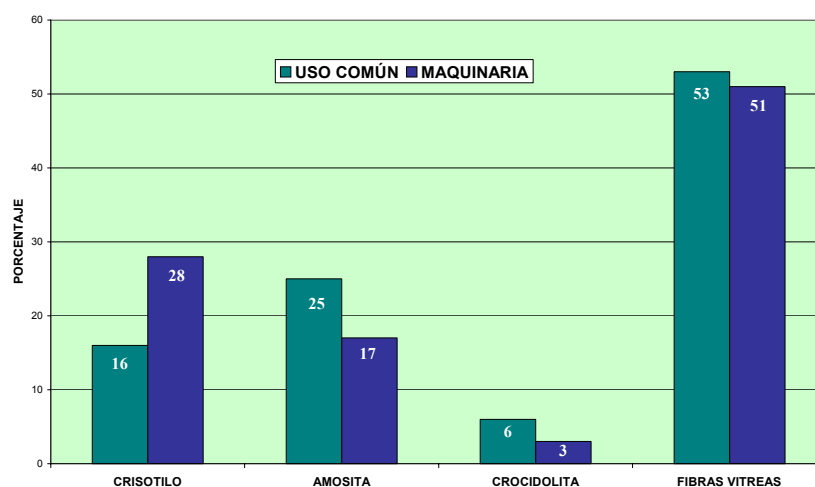
Figura 4. Distribución de los tipos de fibras detectadas en muestras de buques.
