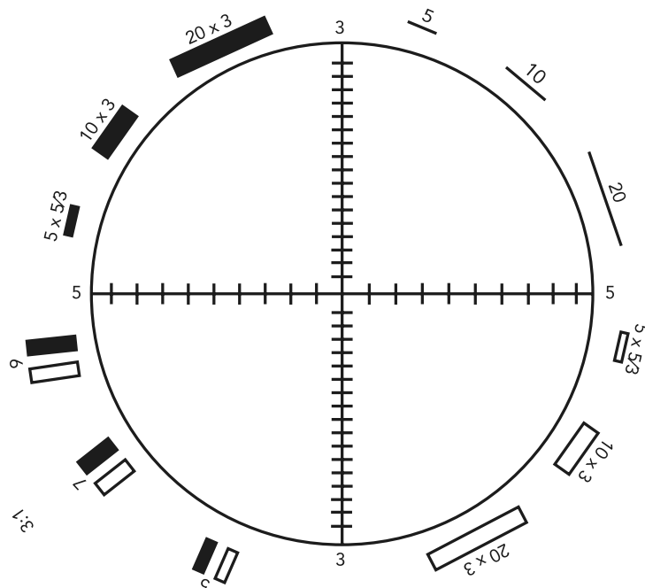
Figura 4. Retículo del ocular de Walton-Beckett del tipo G22.
