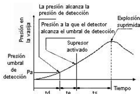
Fig. 2: Secuencia de estadios en el transcurso de una explosión suprimida
