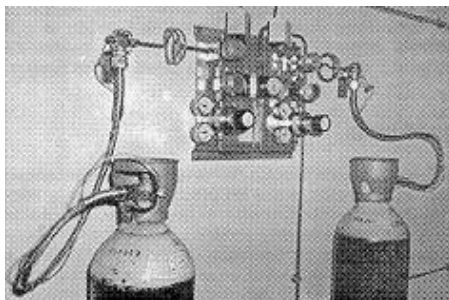
Fig. 4: Cuadro de regulación de presión
