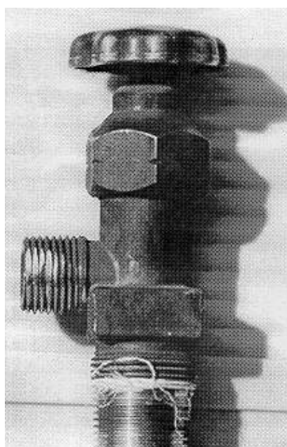
Fig. 6: Grifo de botella con rosca desgastada
