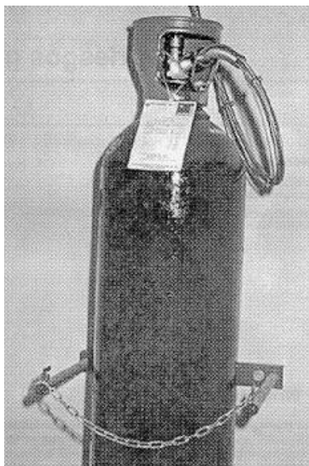
Fig. 3: Botella sujeta con cadena
