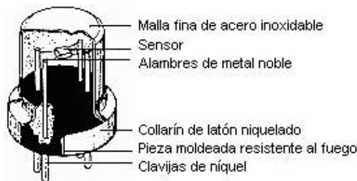
Fig. 4: Detector Taguchi
