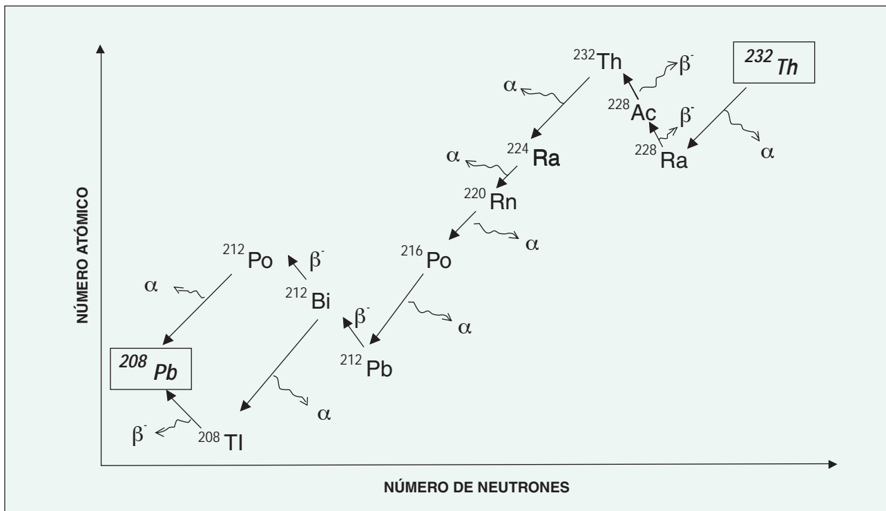
Figura 1. Cadena de desintegración del torio
