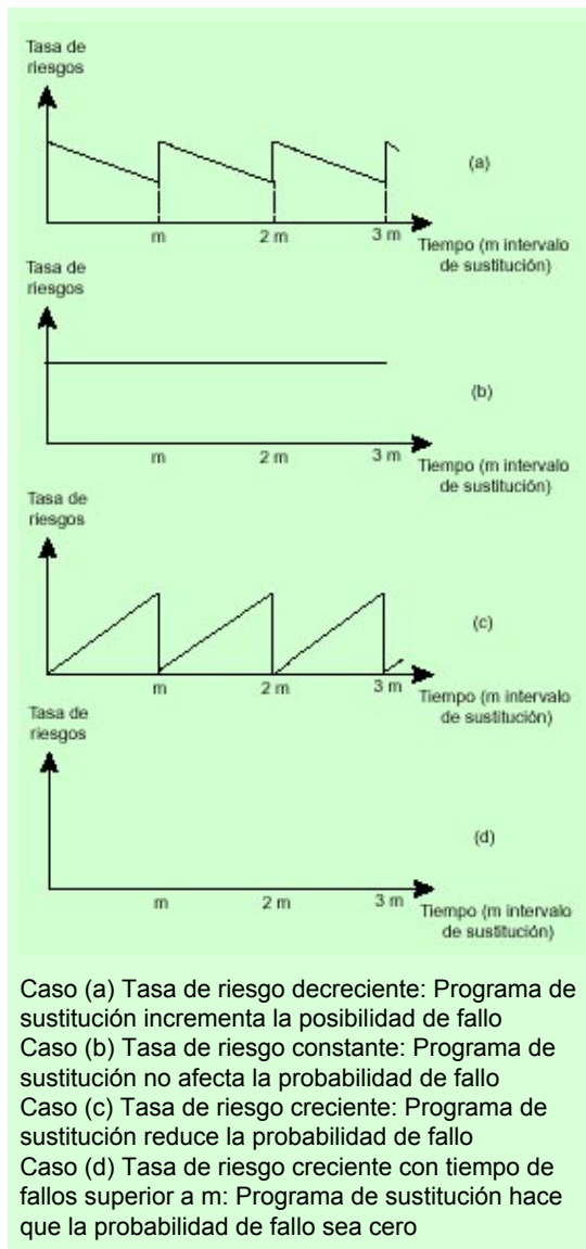
Fig. 1: Relaciones entre la fiabilidad y los programas de sustitución.
